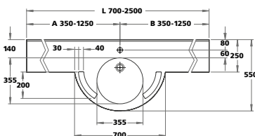
Einzelwaschtisch (Länge ab 700 mm) / Mehrfachwaschtisch (Länge ab 1.550 mm)
