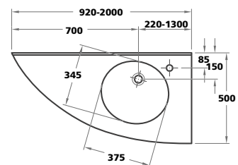
Eckversion (links oder rechts)
