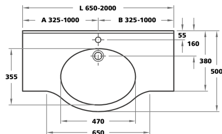
Einzelwaschtisch (Länge ab 650 mm) / Mehrfachwaschtisch (Länge ab 1.300 mm)
