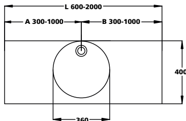
Einzelwaschtisch (Länge ab 600 mm) / Mehrfachwaschtisch (Länge ab 1.200 mm)
